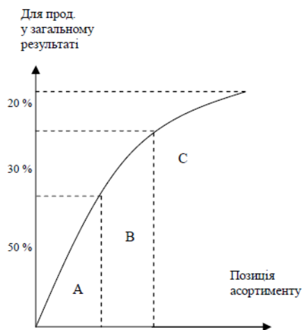
Рис. 1. ABC-аналіз[3]
